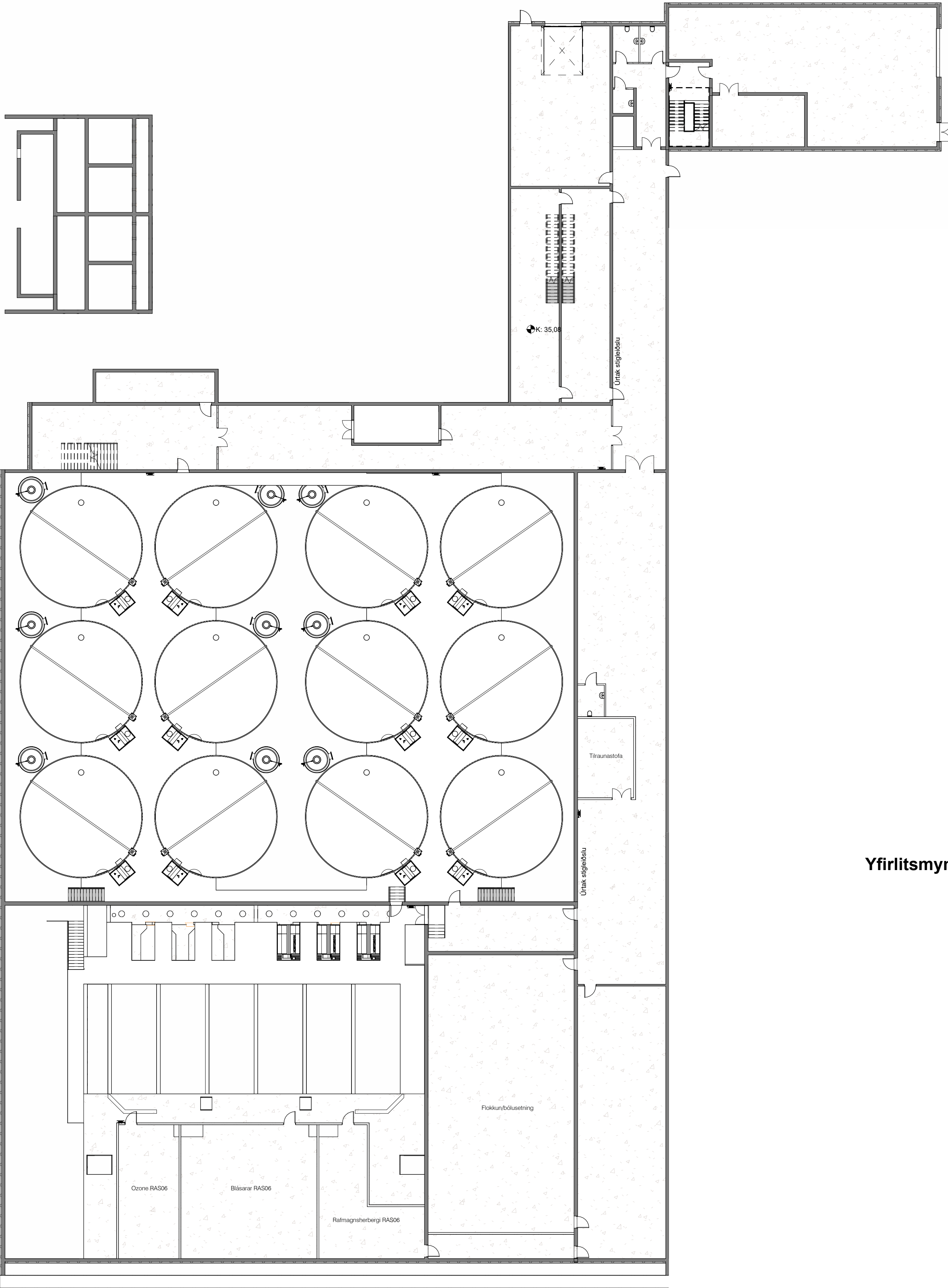
Yfirlitsmynd 2. hæðar
