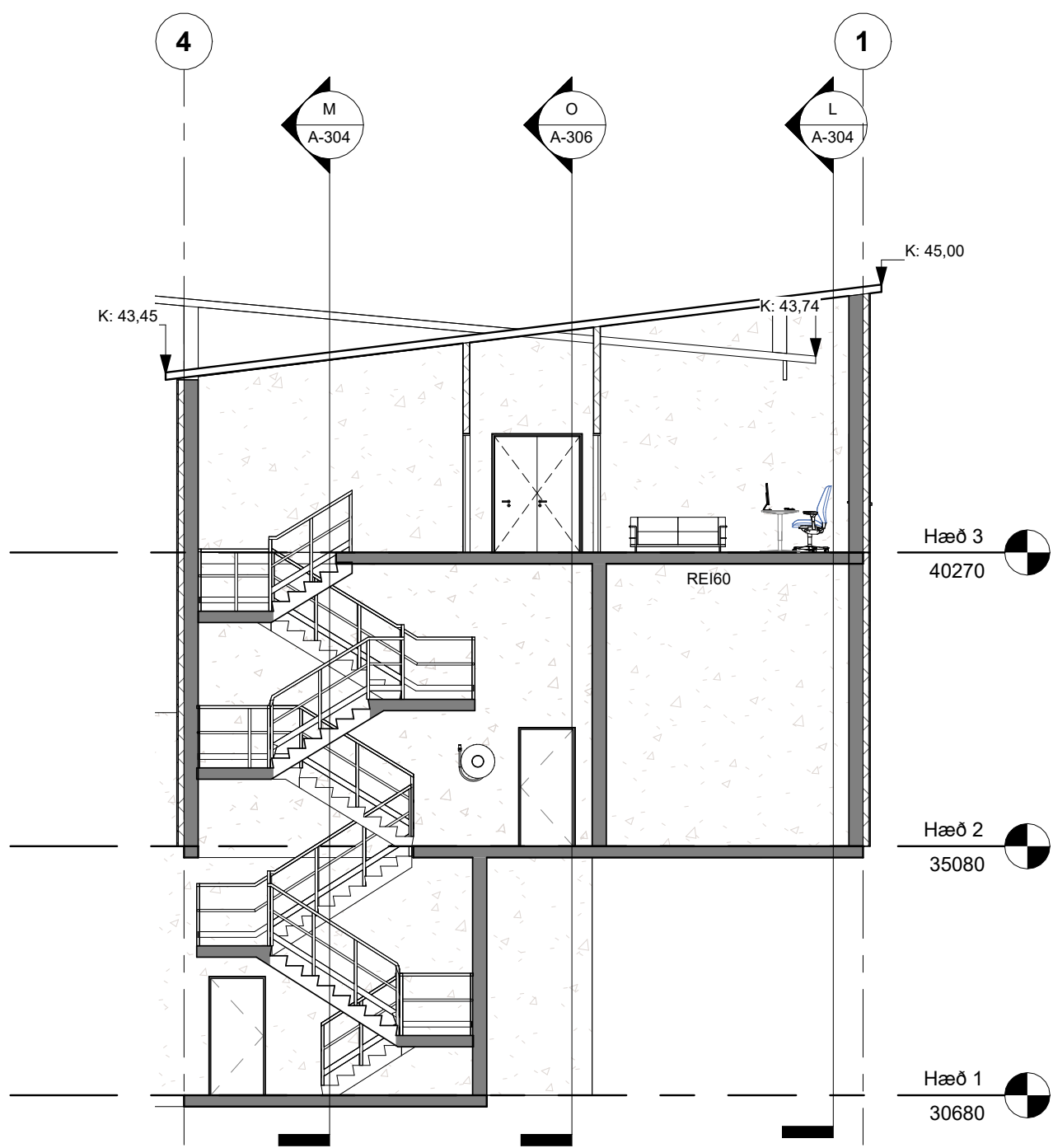
Sneiðing A-A mkv: 1 : 100
