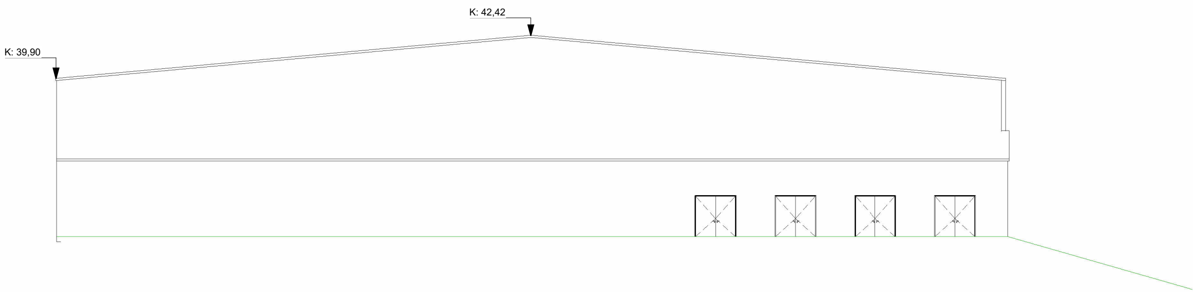
Útlit - Surður-Vestur mkv: 1 : 200
