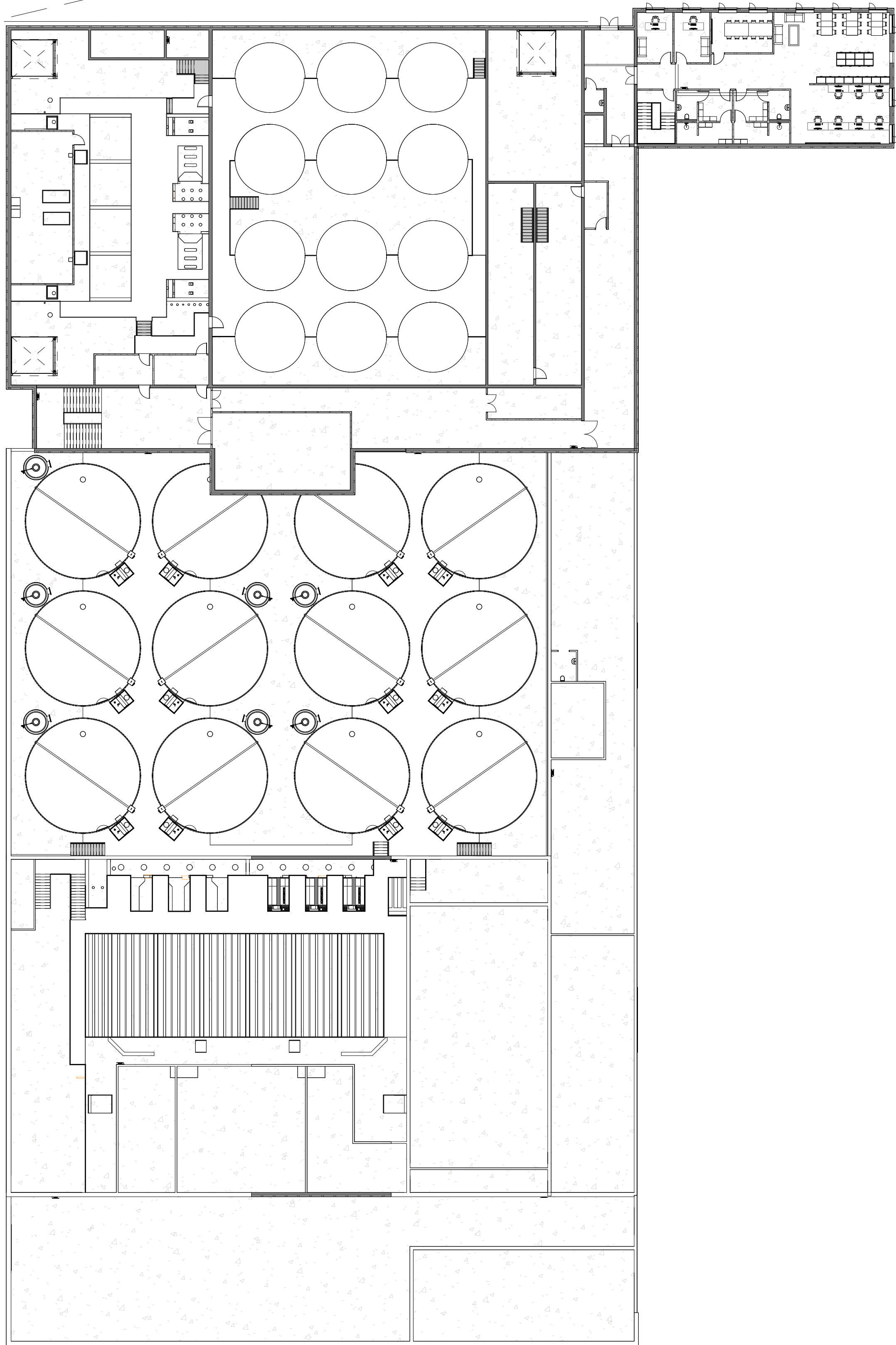
Yfirlitsmynd 1 : 250
