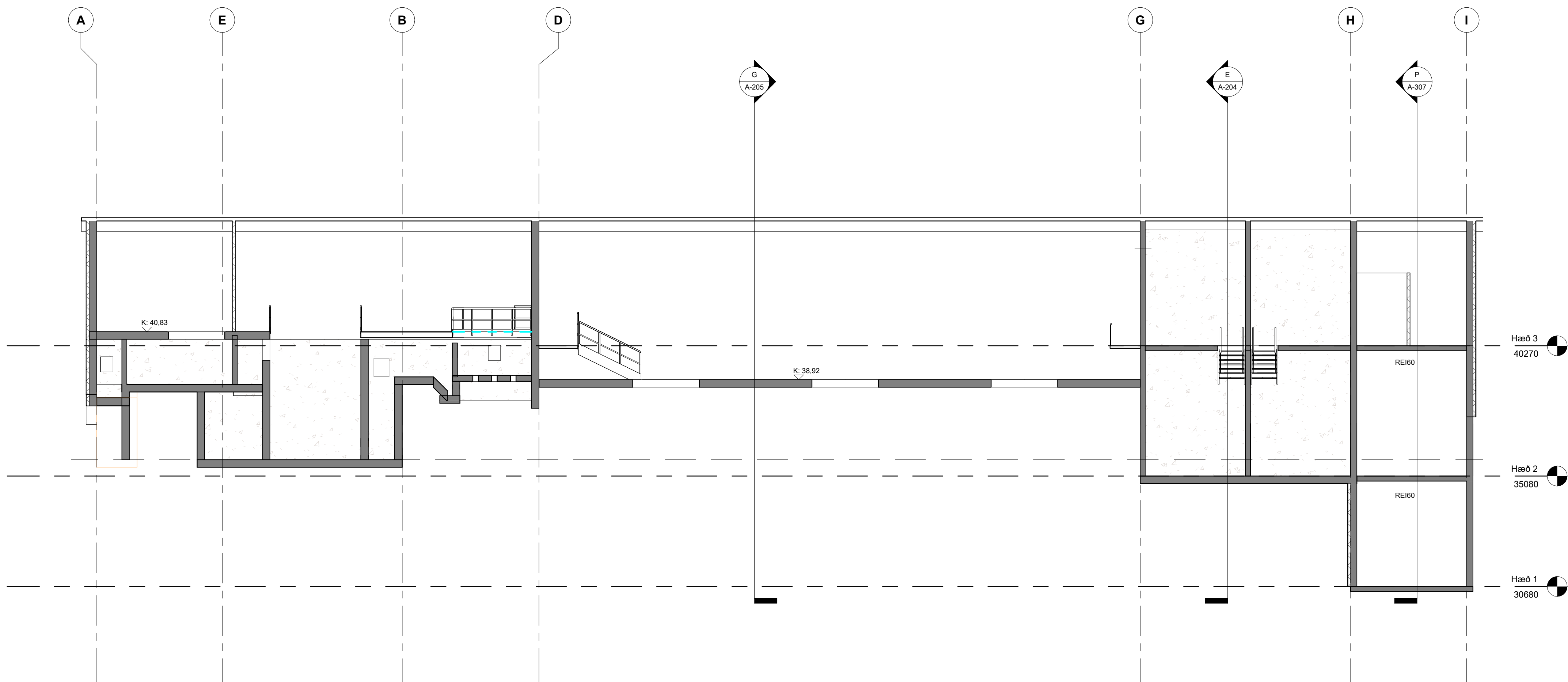
Sneiðing N-N mkv: 1 : 100
