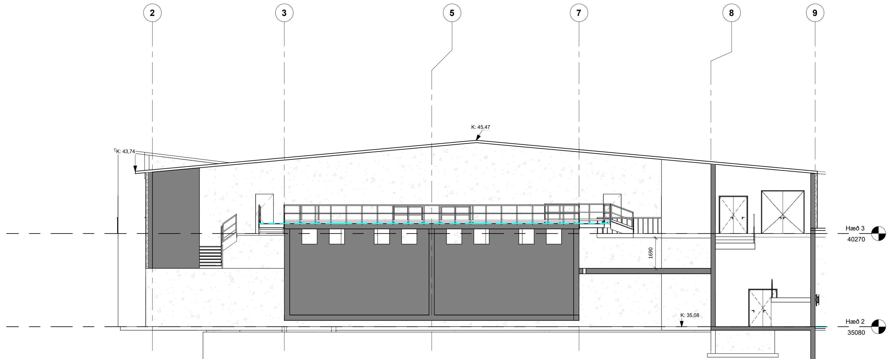
Sneiðing F-F mkv: 1 : 100
