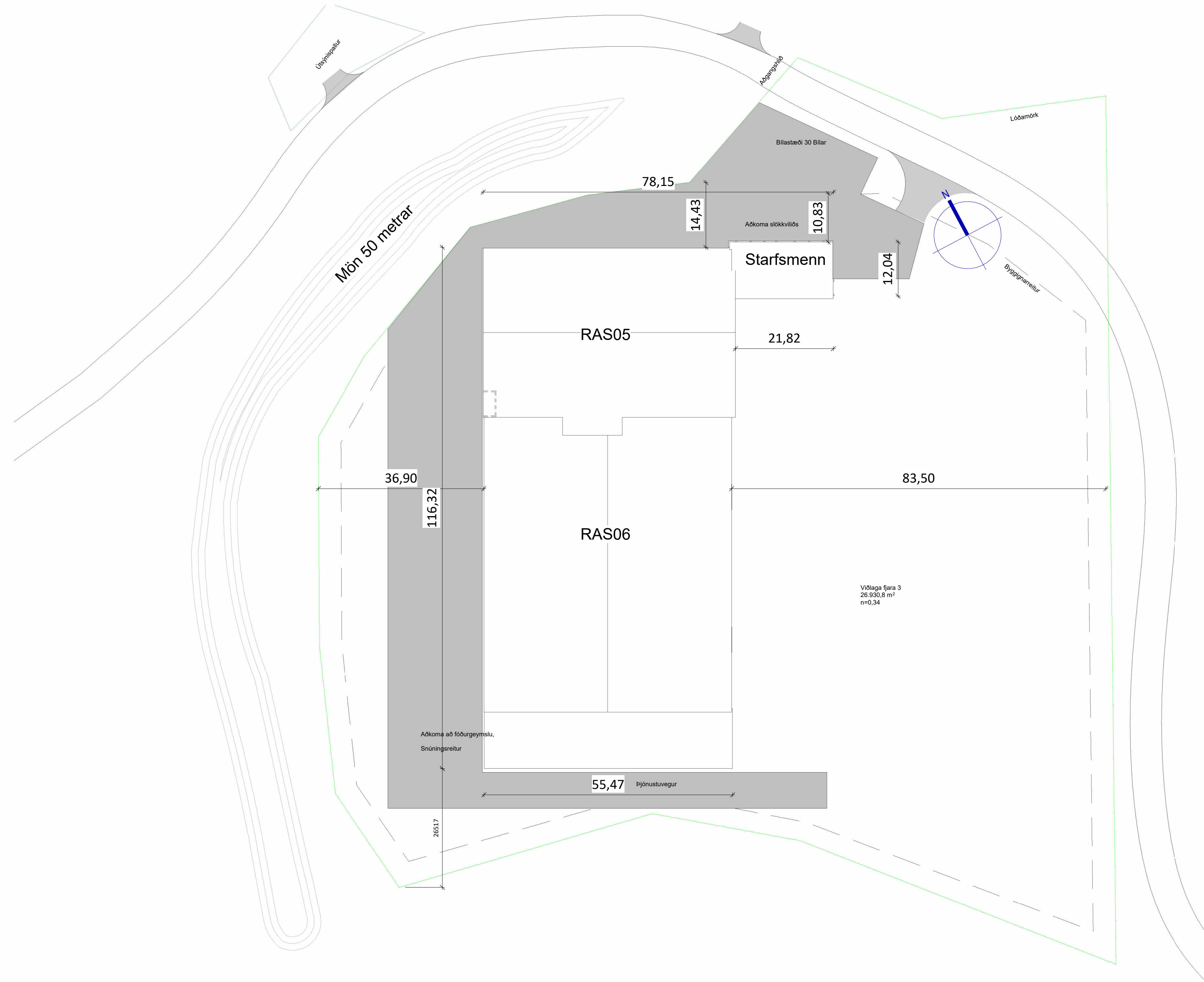
Afstöðumynd 1 : 500
