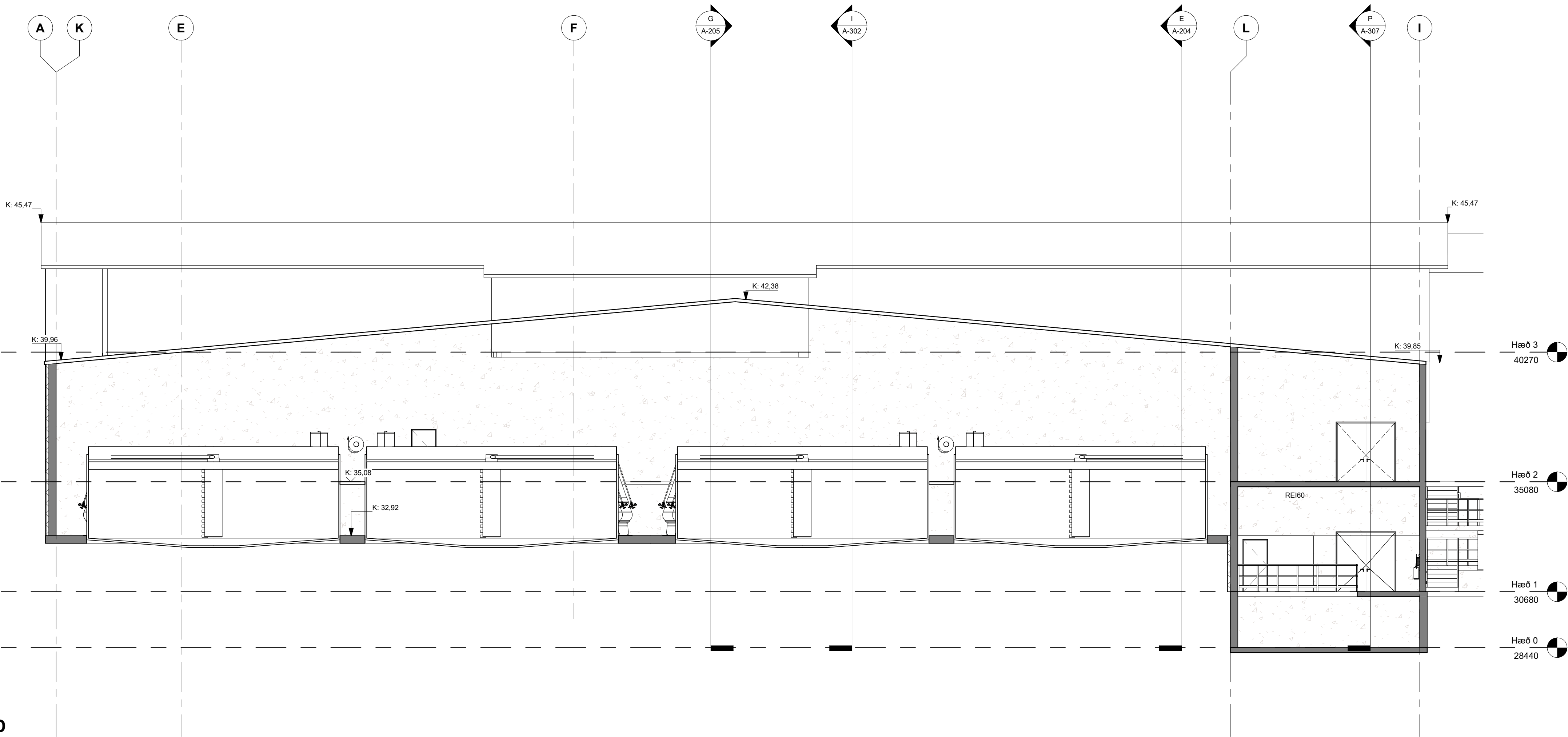
Sneiðing D-D mkv: 1 : 100
