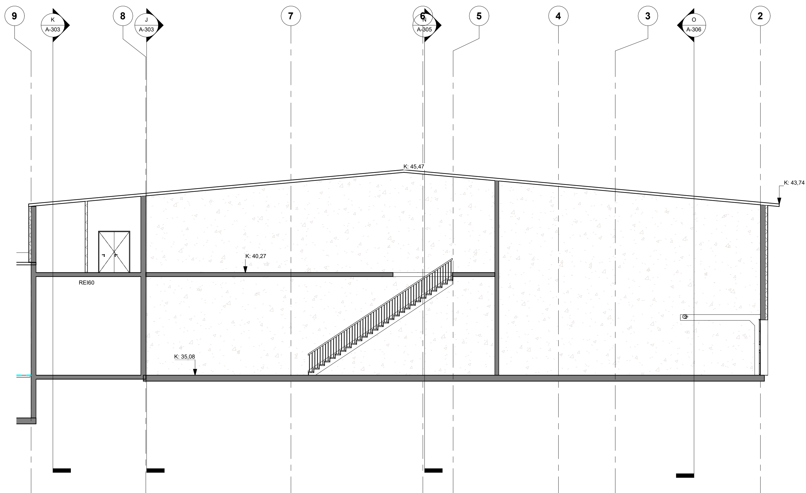
Sneiðing E-E mkv: 1 : 100
