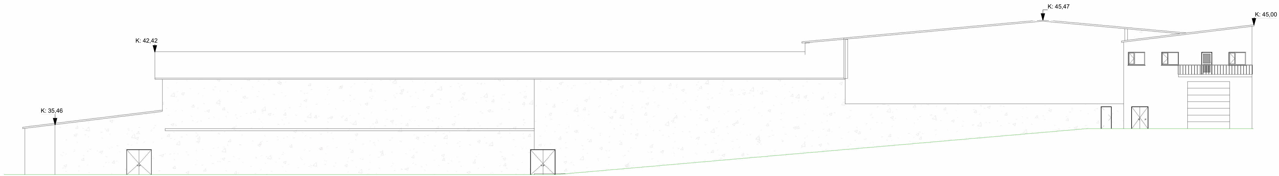
Útlit - Austur-Surður mkv: 1 : 200
