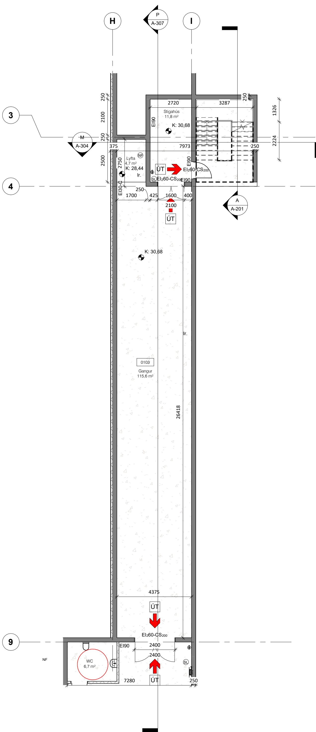
Grunnmynd 1. hæðar - Svæði 3 1 : 100
