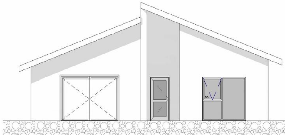
Norðurhlið 1 : 100
